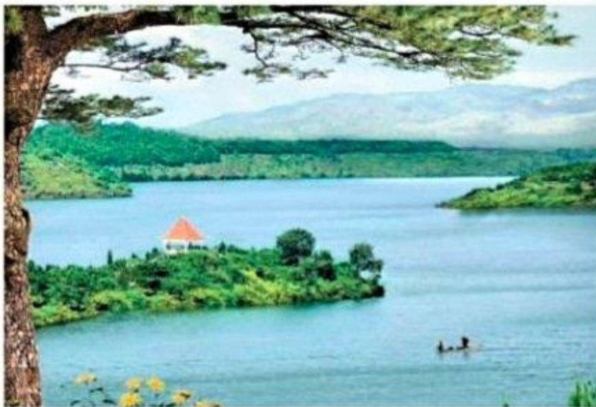
Hình 17.3. Hồ Tơ Nưng (T'Nưng) ở thành phố Plây-ku (Pleiku), Gia Lai (Việt Nam) được hình thành từ miệng núi lửa đã tắt
