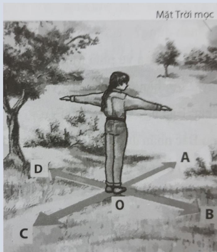
Hình 8.1. Xác định phương hướng bằng quan sát Mặt Trời mọc
